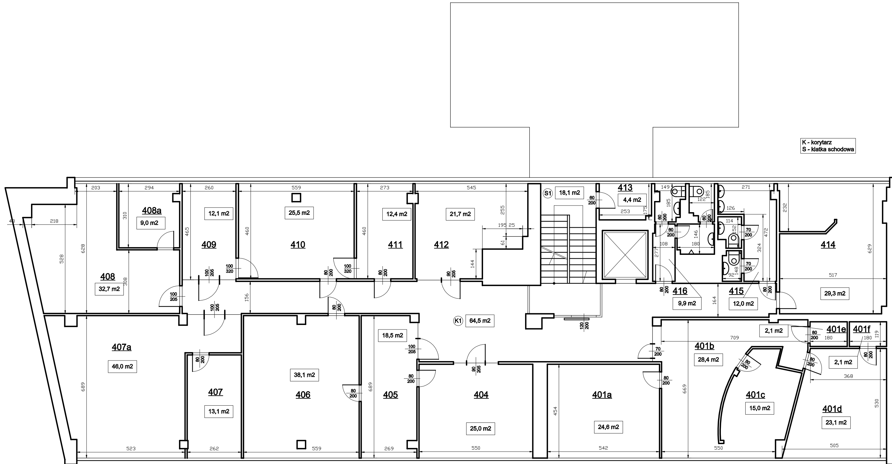
Rzut 3 piętra skala 1:110 Rys. 5
