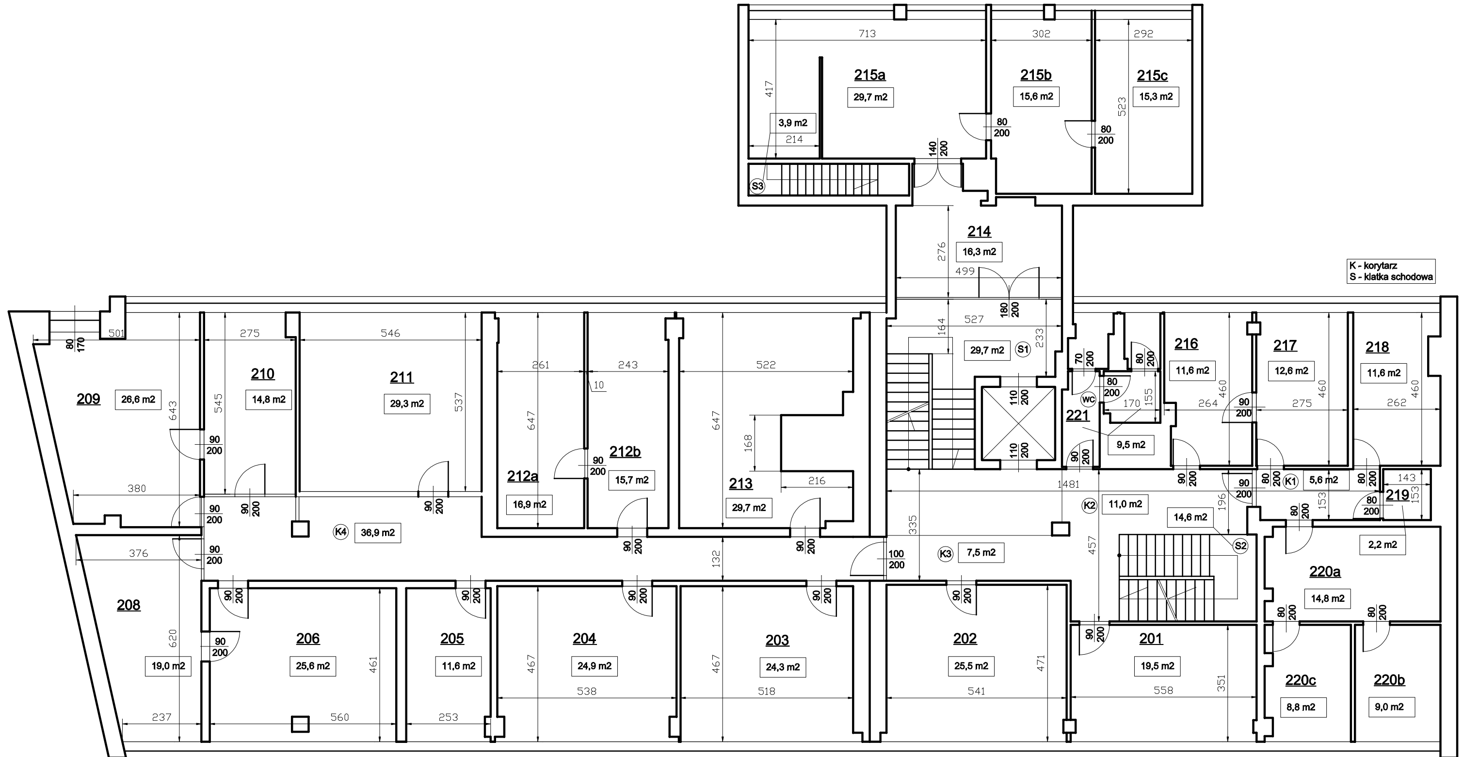
Rzut 1 piętra skala 1:110 Rys. 3
